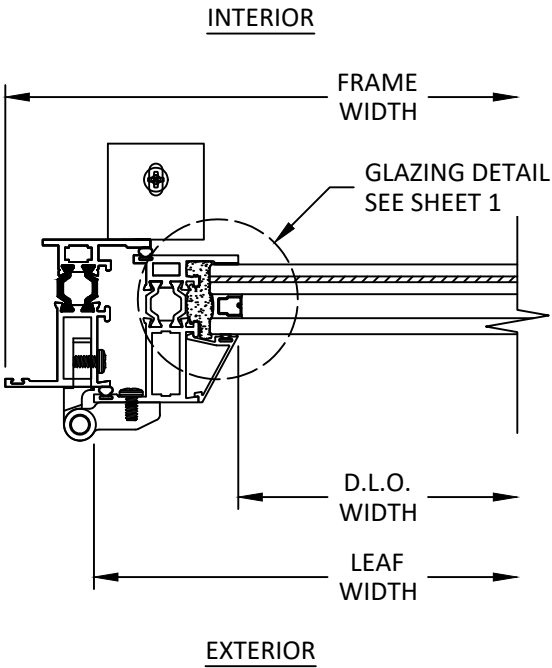
D 6 HORIZONTAL SECTION HINGE JAMB
